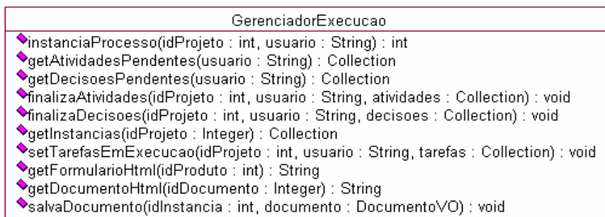
Fig. 4-19 - Classe GerenciadorExecucao
