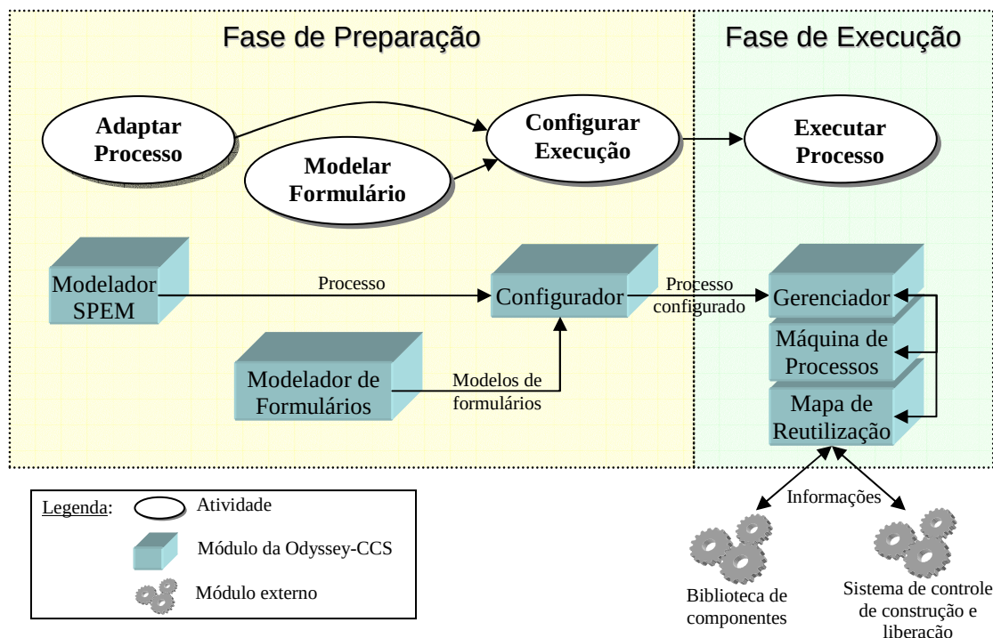
Fig. 3-1 - Abordagem Odyssey-CCS
