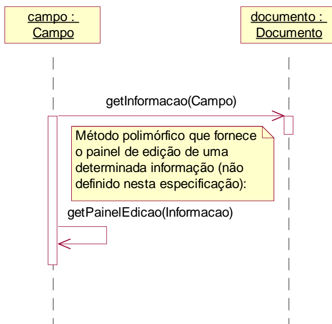
Figura A.25: Diagrama de seqüência do método getPainelEdicao(Documento documento)
