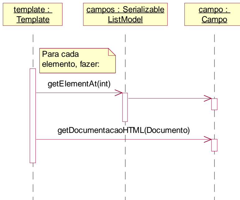
Figura A.31: Diagrama de seqüência do método getElementAt(int)
