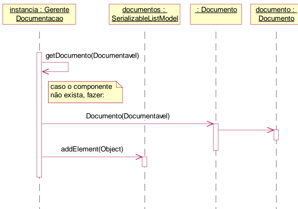
Figura A.1: Diagrama de seqüência do método addComponente(Documentavel componente)
