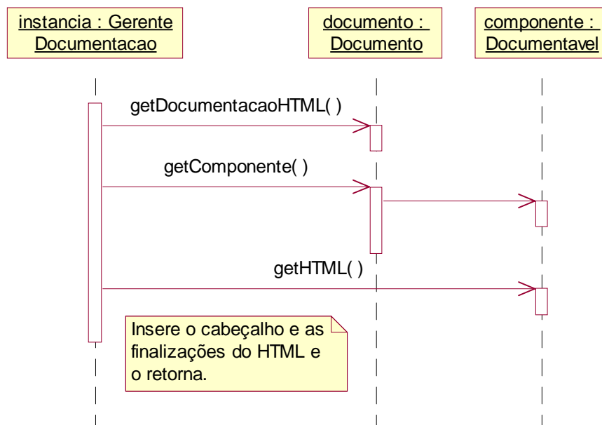
Figura A.28: Diagrama de seqüência do método getDocumentacaoHTML(Documento documento)
