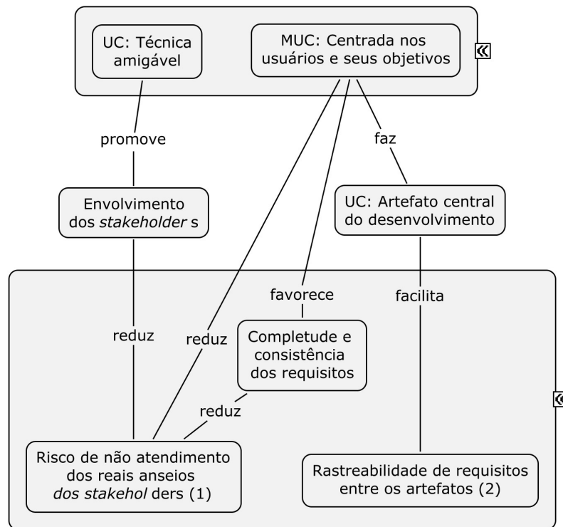
Figura 2.3 – Características da MUC e vantagens em relação à LRqs
