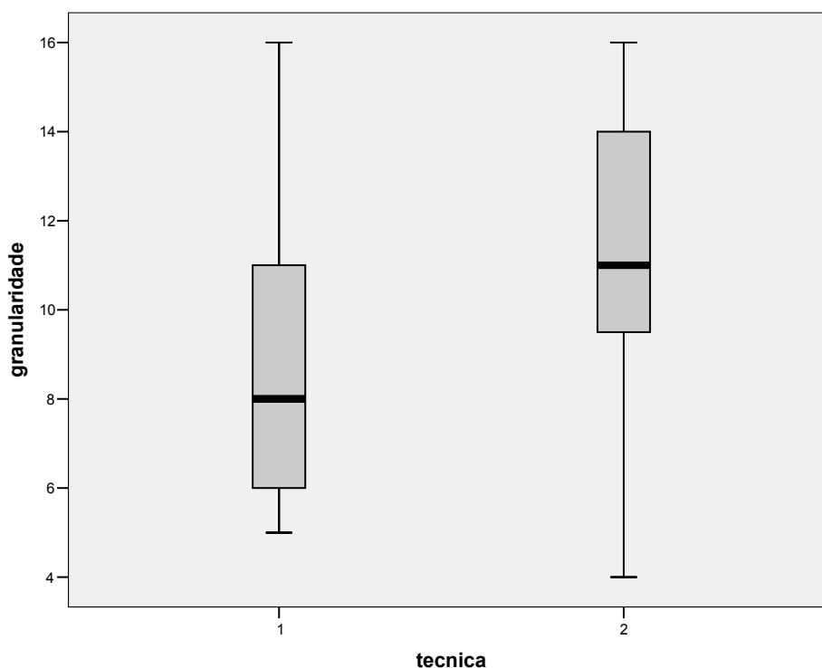
Figura 6.2 – Diagrama Box-Plot para a variável Granularidade
