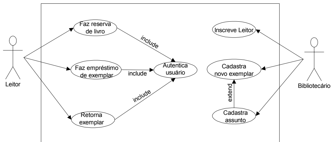
Figura 2.1 – Diagrama de UCs
