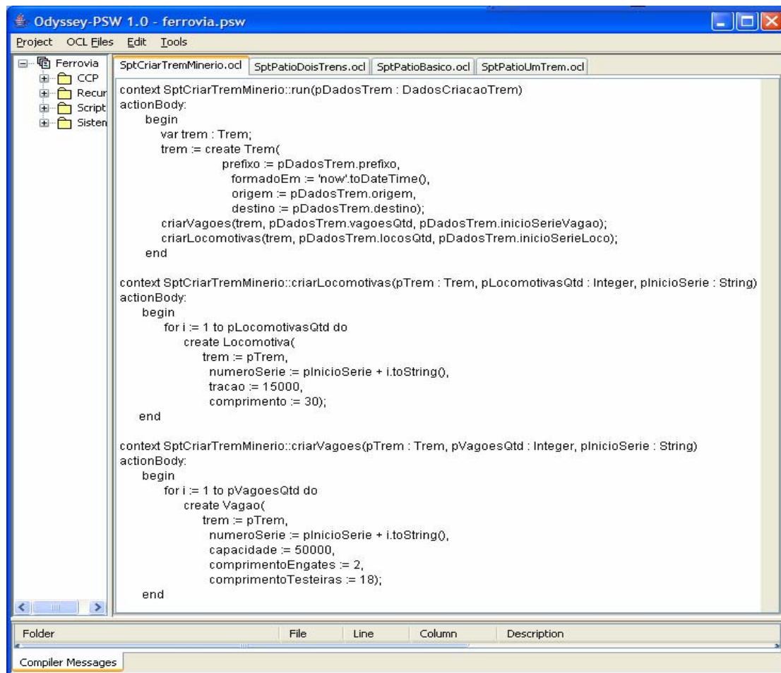
Figura 8.12 - Script de criação de um trem de minério
